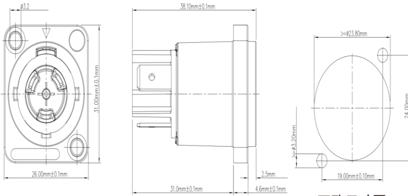
开孔尺寸图
