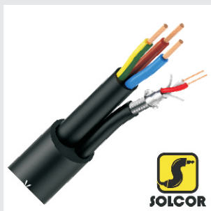
Cable Híbrido DMX & Poder Código: CHDXPOW Calibre Cable Poder: 3x14 AWG Calibre Cable DMX: 2X22 AWG, (OFC) Diámetro Exterior: 17 mm Color: Negro Presentación: Carrete 100 mts.
